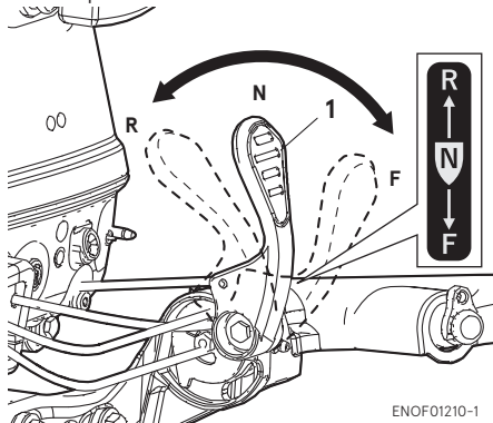
1. Levier inverseur
